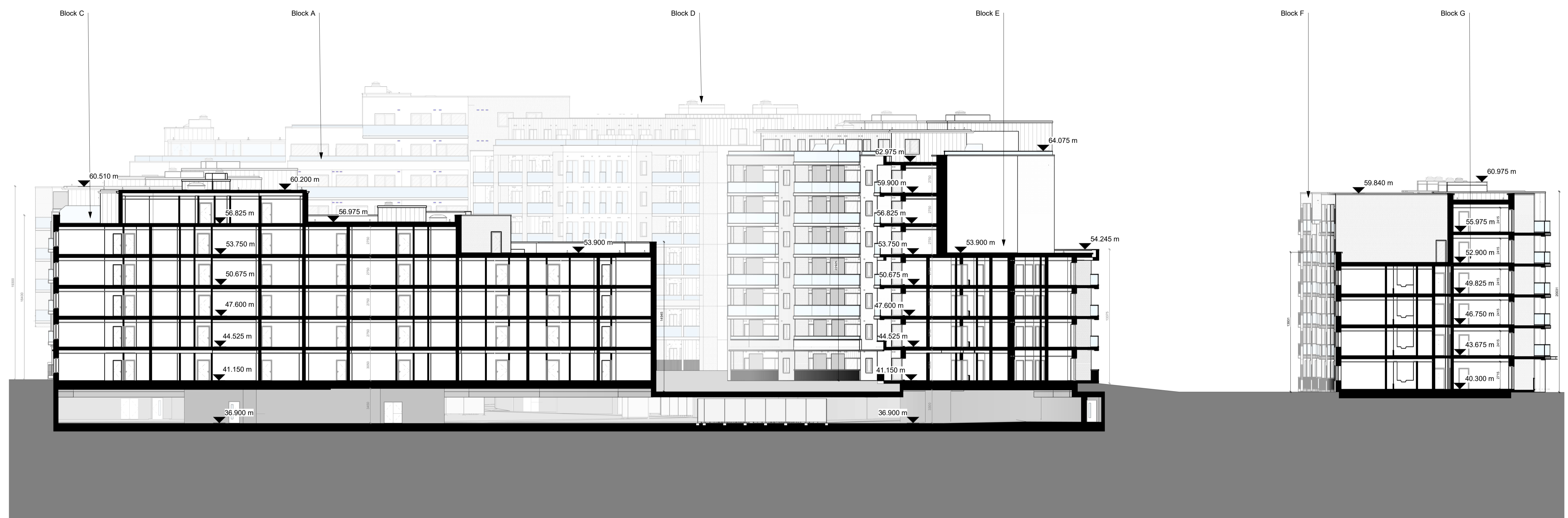
1 Section BB 1:200
